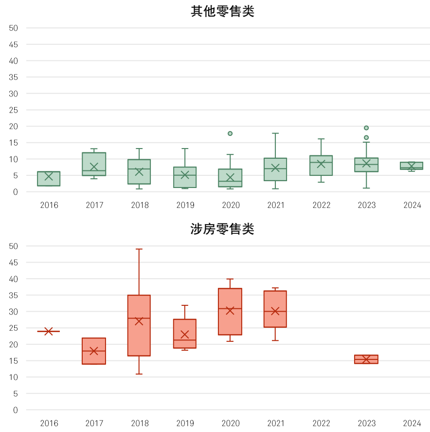
图表8：历年各类不良ABS产品优先级证券到期期限（月）
