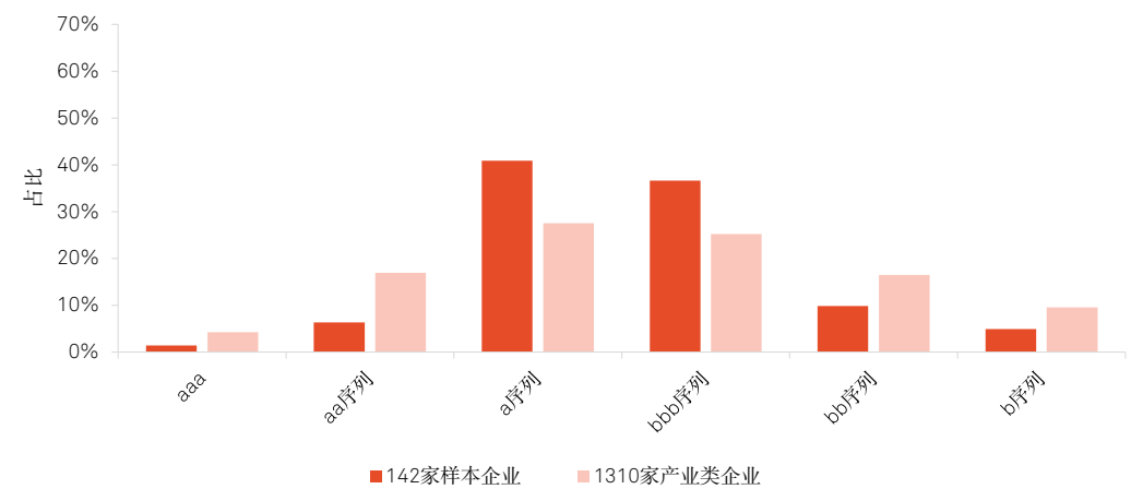
样本企业在个体信用状况层面与传统产业类发行人的差距不大
