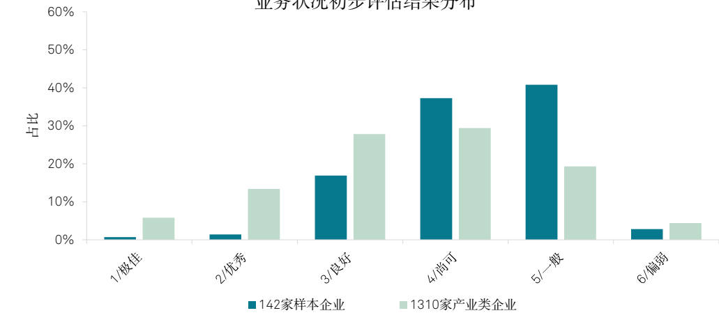
相比于传统产业类发行人，可转债发行人的业务状况普遍较弱 业务状况初步评估结果分布
