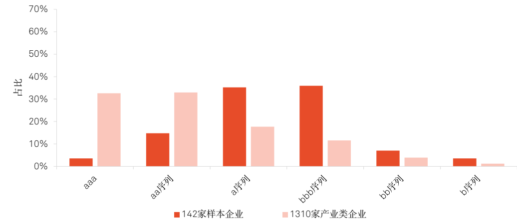
可转债发行人的主体信用质量明显弱于传统产业类发行人
