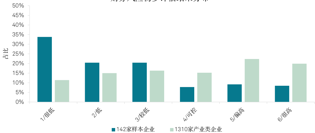
相比于传统产业类发行人，可转债发行人的财务风险普遍不高 财务风险初步评估结果分布
