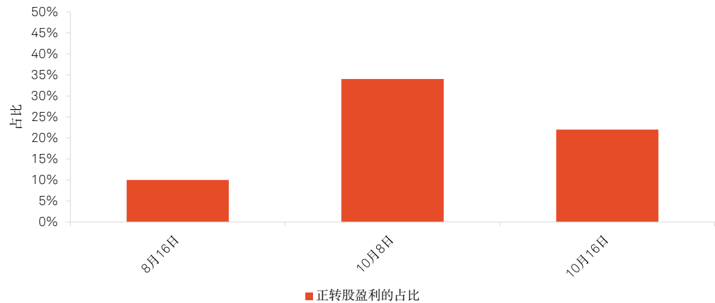
图9 142家样本企业其转股盈利性普遍较弱 样本企业存续可转债有转股正盈利的占比
