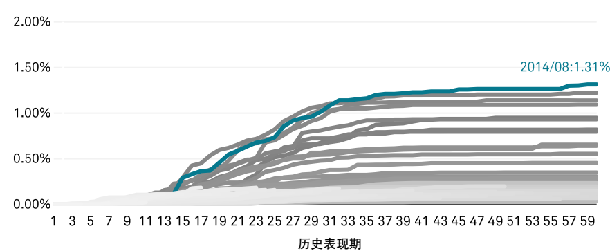
图表 18 静态池分析—历史累计核销率
