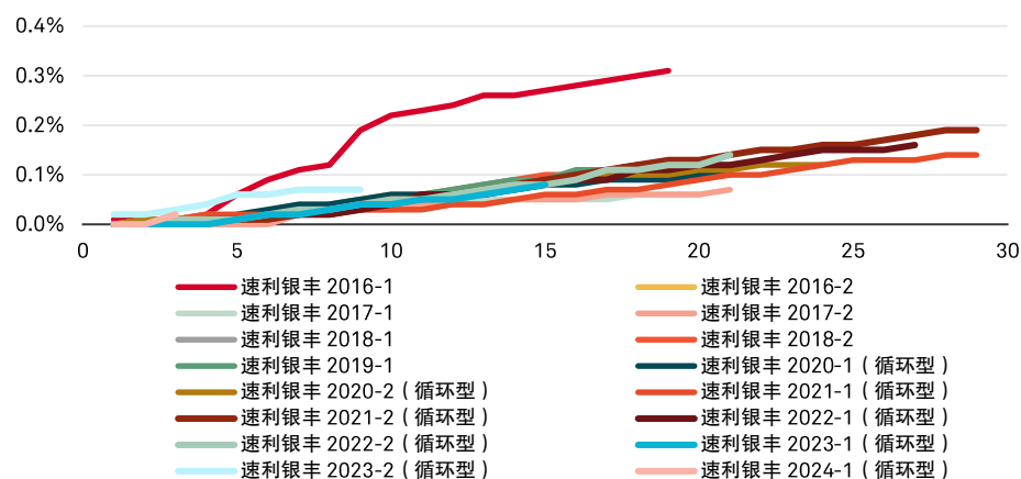
图表 4 奔驰汽车金融已发行项目累计违约率
