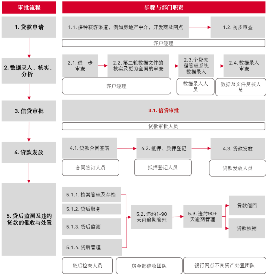
图表 5 建设银行个贷流程管理系统（PLPM）全流程
